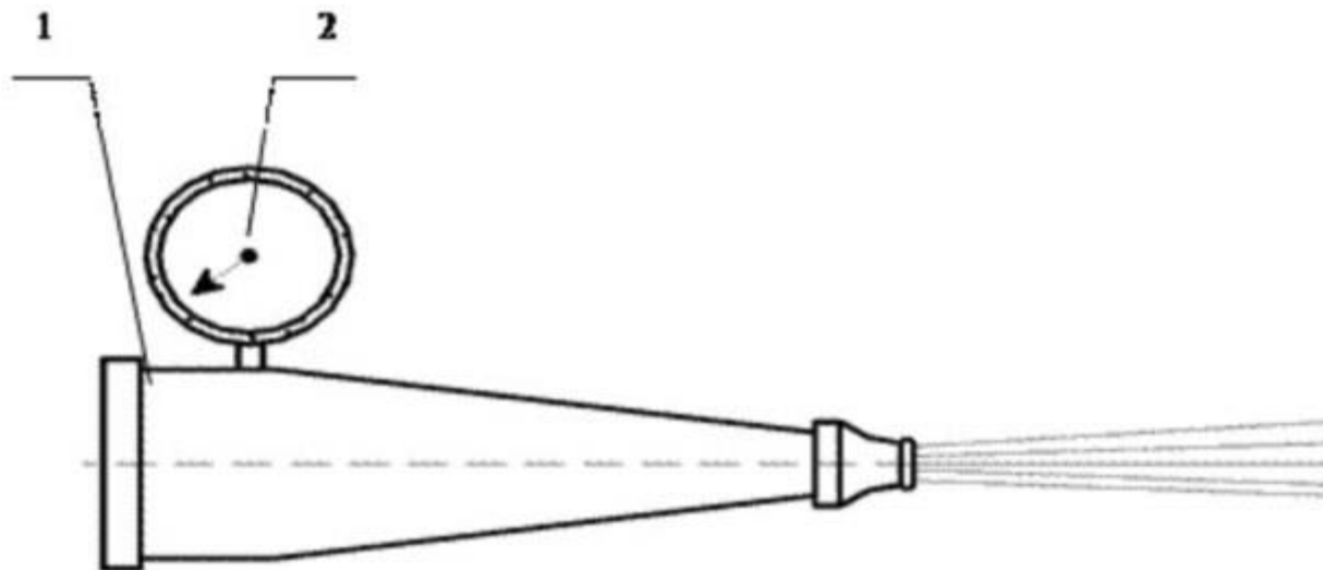
Схема ствола-водомера
